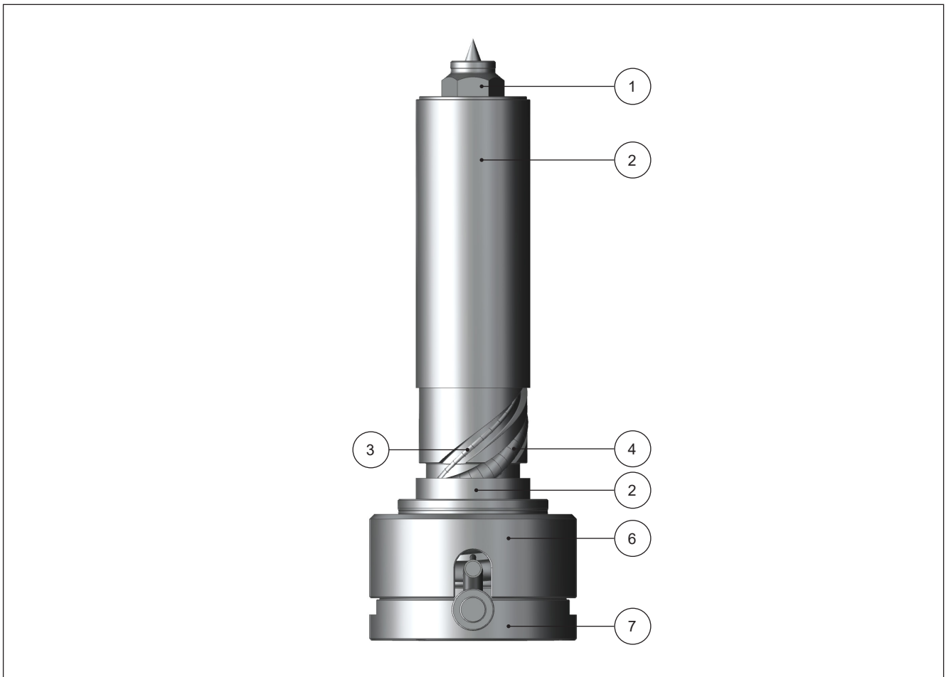
Abbildung 86: HPS III Düse für Standardmontage
