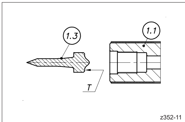
Abbildung 66: Düsen Spitze montieren
