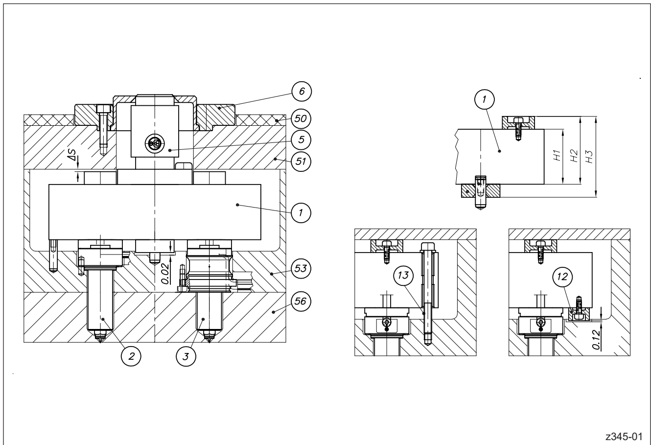
Abbildung 23: Prinzipieller Aufbau eines Systems mit HPS III-S / pro SHOT Düsen für Standard- und Frontmontage
