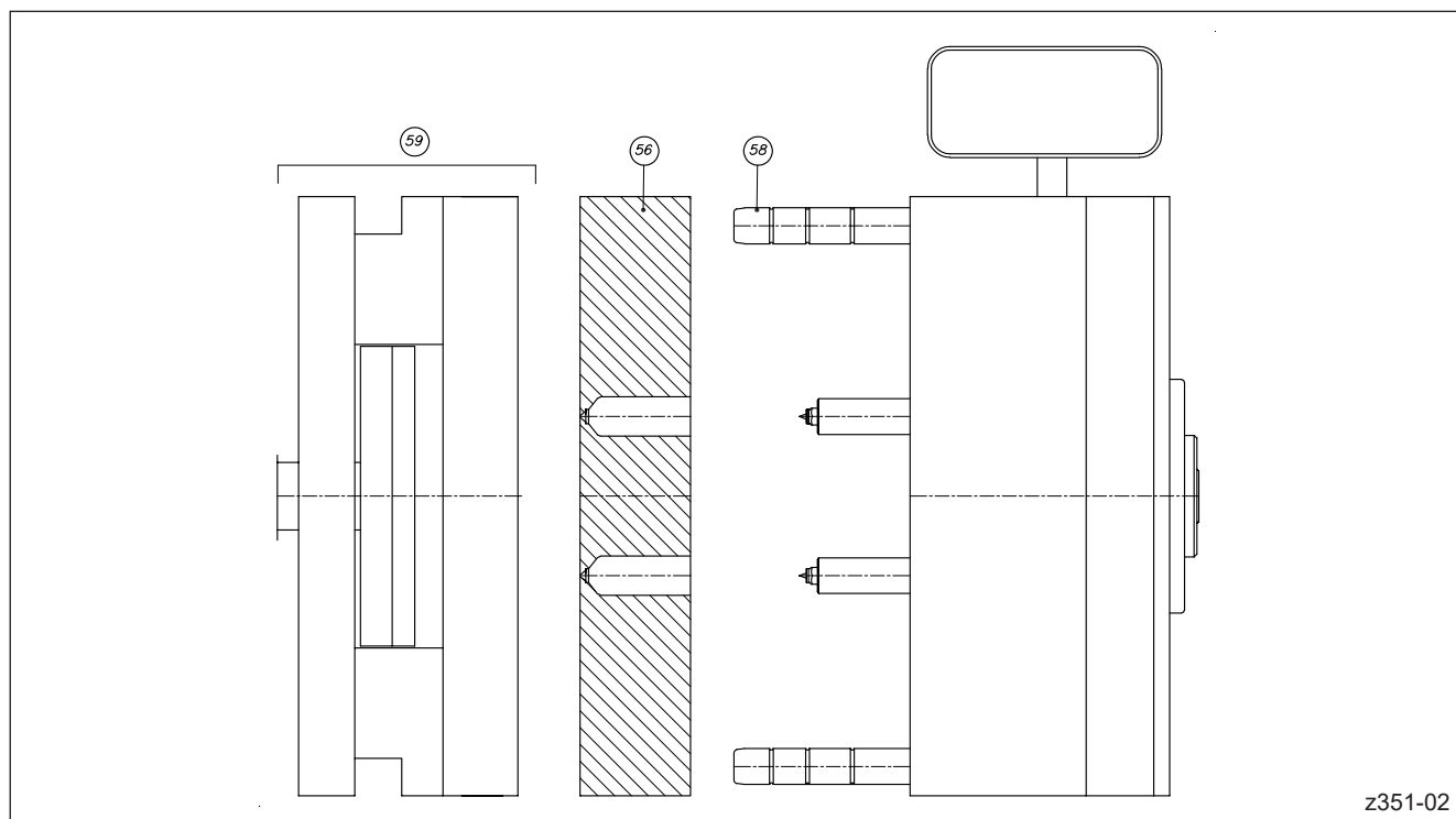
Abbildung 41: Montagevorgang
