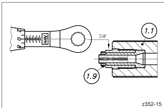
Abbildung 60: Düsenspitze anziehen
