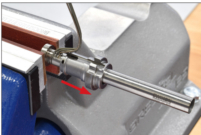
Abbildung 73: Düsenkörper abziehen
