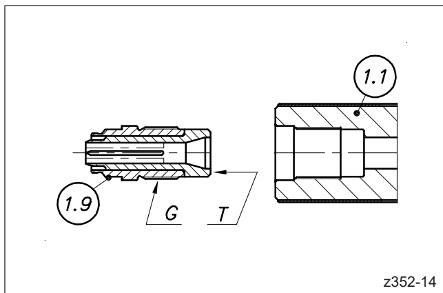
Abbildung 59: Düsenspitze montieren
