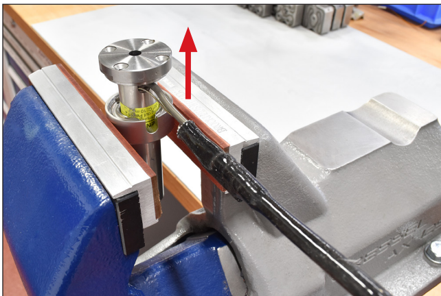
Abbildung 89: Druckrohr herausziehen
