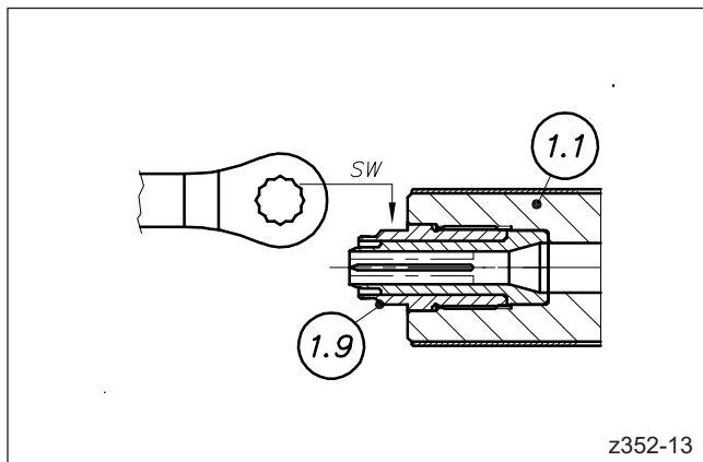
Abbildung 58: Düsenspitze herauserschrauben
